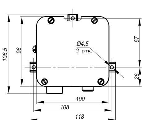
Рис. 6 Присоединительные размеры датчика в силуминовом корпусе
