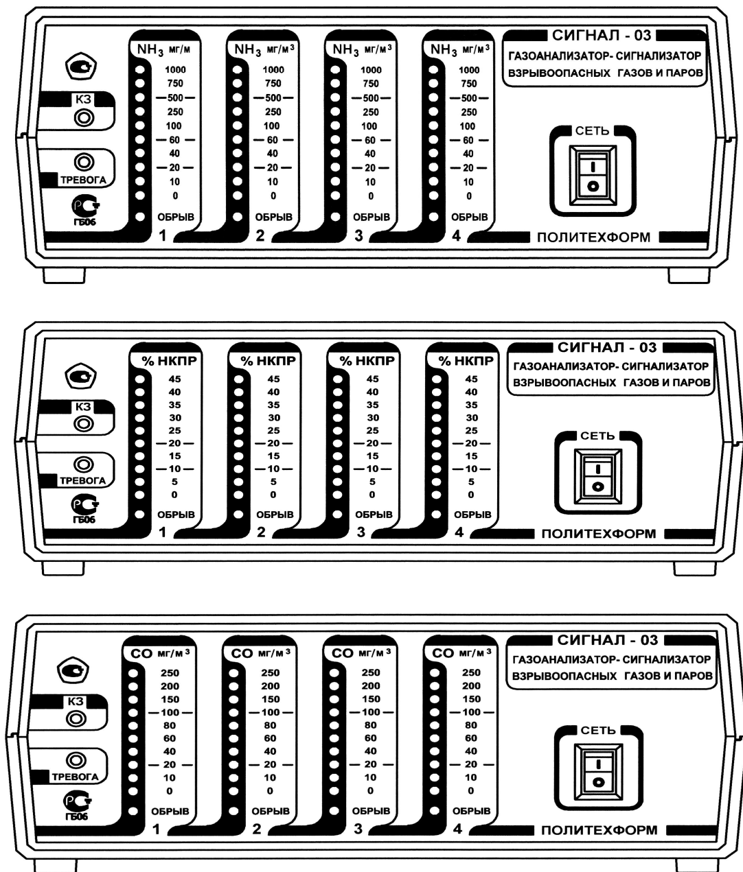
Рис.1. Внешний вид блока информационного Сигнал-03.БИ с линейными светодиодными шкалами на пары аммиака, ВОГ и оксид углерода
