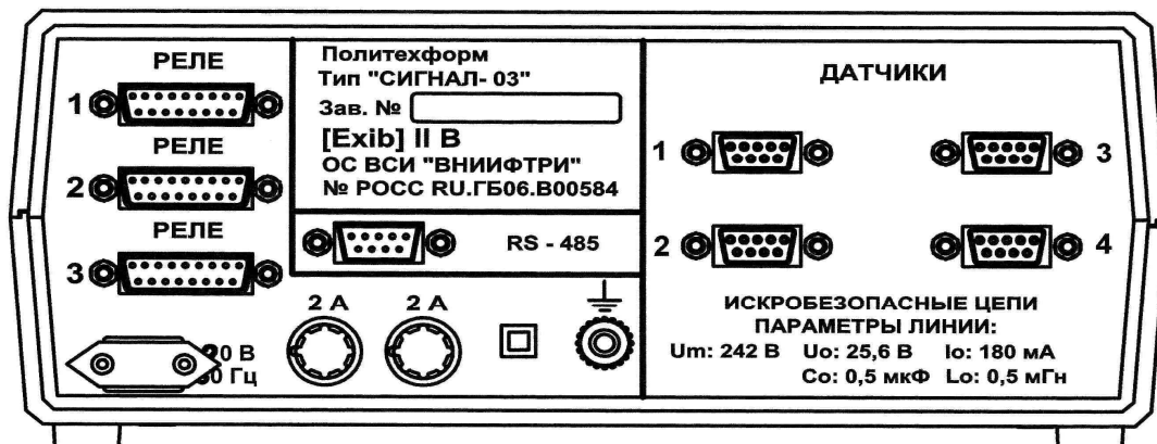
Рис.2. Вид задней панели блока информационного
