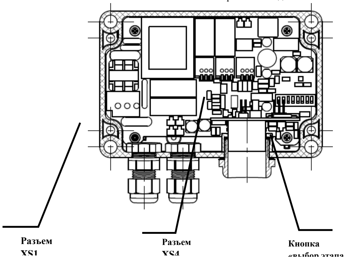
Рисунок А.1 — Расположение клемм подключения к колодкам питания на плате силовой
