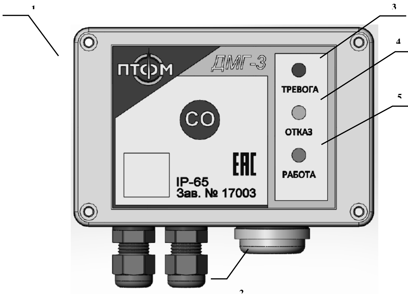
Рисунок 2 — Передняя панель детектора
