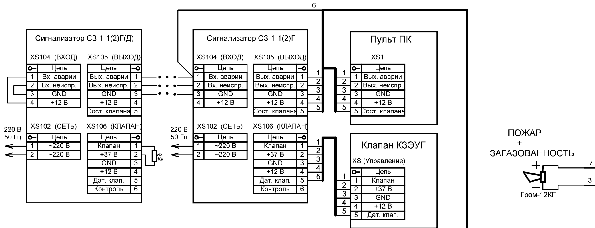
Приложение к паспорту БППИ УС ЯБКЮ421453.027 ПС Подключение ИП212-45 к системе САКЗ-МК-1
