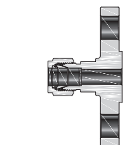
Фланцевый переходник
