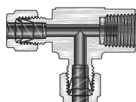
Тройник с внутренней резьбой сбоку
