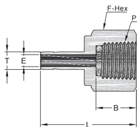
1" и меньше
