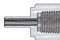
Трубный адаптер с внутренней резьбой
