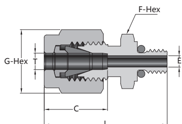
Дюймовая трубка
