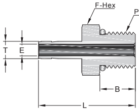
1" и меньше
