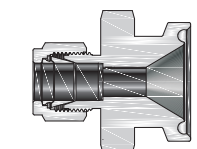
Переходник с санитарного фланца
