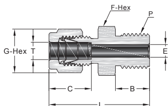
Дюймовая трубка
